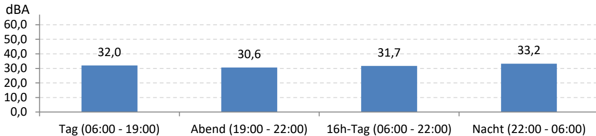
Abb. 6: LEQ für den gesamten Messzeitraum während der Messdauer (Gesamt: 888 Stunden)
