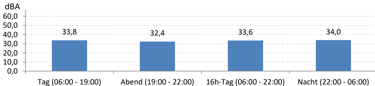
Abb. 7: LEQ bei Pistenbetriebsrichtung "westliche Winde" 543 Stunden im Messzeitraum
