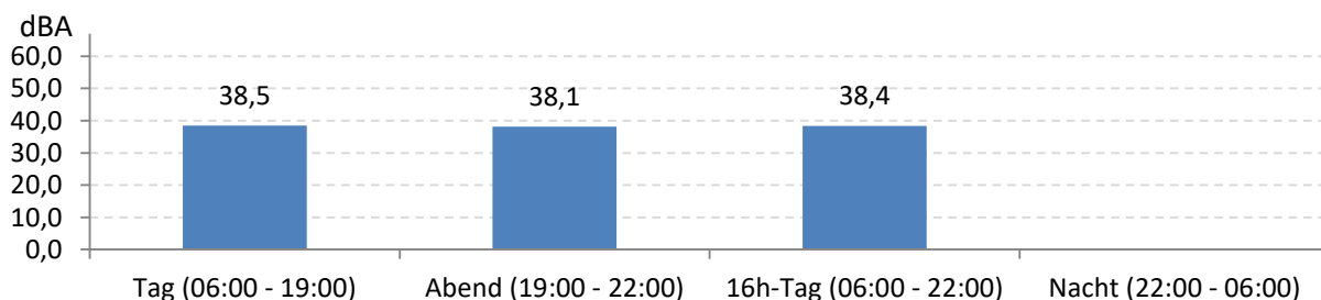
Abb. 9: LEQ bei Pistenbetriebsrichtung "östliche Winde" 78 Stunden im Messzeitraum
