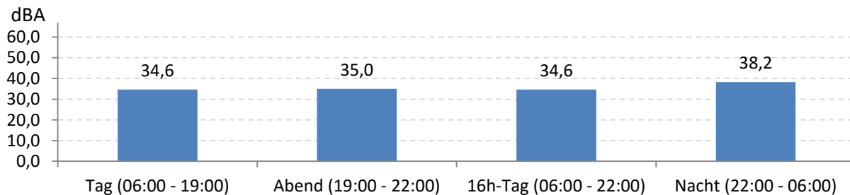
Abb. 7: LEQ bei Pistenbetriebsrichtung "westliche Winde" 519 Stunden im Messzeitraum
