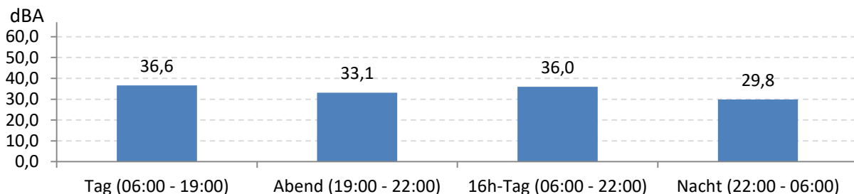
Abb. 8: LEQ bei Pistenbetriebsrichtung "Windstille" 243 Stunden im Messzeitraum
