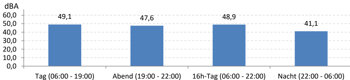
Abb. 7: LEQ bei Pistenbetriebsrichtung "westliche Winde" 367 Stunden im Messzeitraum
