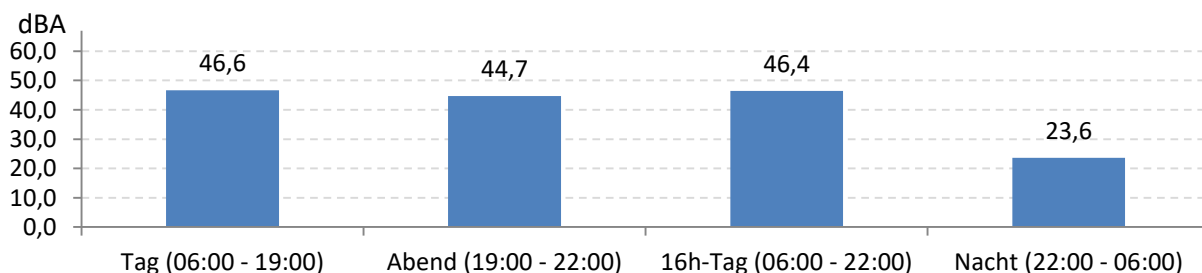
Abb. 9: LEQ bei Pistenbetriebsrichtung "östliche Winde" 155 Stunden im Messzeitraum
