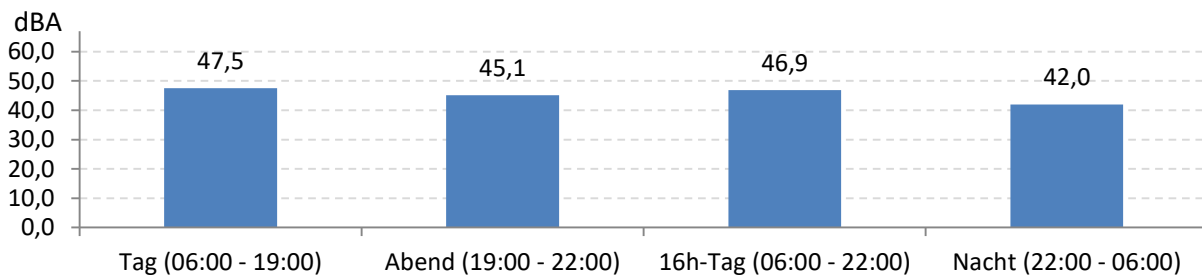
Abb. 8: LEQ bei Pistenbetriebsrichtung "Windstille" 174 Stunden im Messzeitraum
