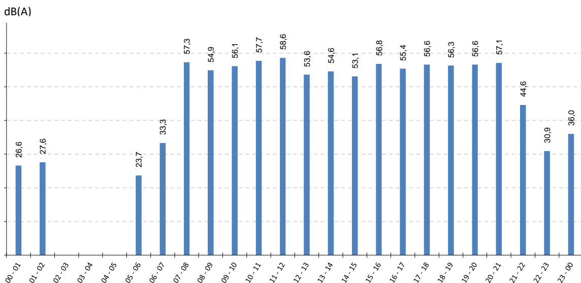
Abb. 11: Verlauf der über den Meßzeitraum gemittelten Stunden-LEQs für Flugverkehr
