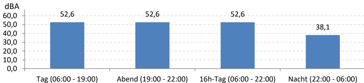
Abb. 7: LEQ bei Pistenbetriebsrichtung "westliche Winde" 403 Stunden im Messzeitraum
