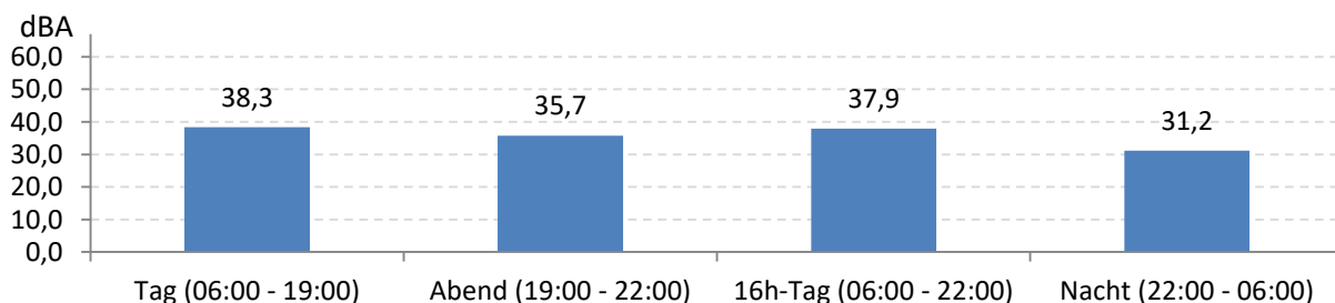
Abb. 9: LEQ bei Pistenbetriebsrichtung "östliche Winde" 228 Stunden im Messzeitraum
