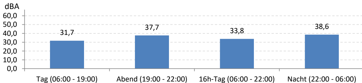
Abb. 7: LEQ bei Pistenbetriebsrichtung "westliche Winde" 423 Stunden im Messzeitraum
