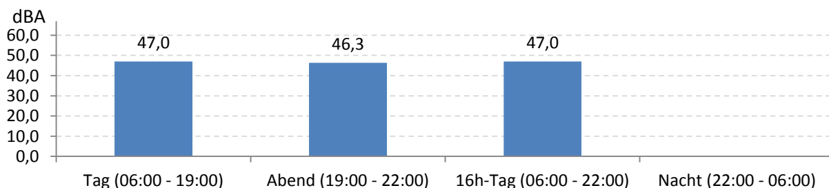
Abb. 9: LEQ bei Pistenbetriebsrichtung "östliche Winde" 47 Stunden im Messzeitraum
