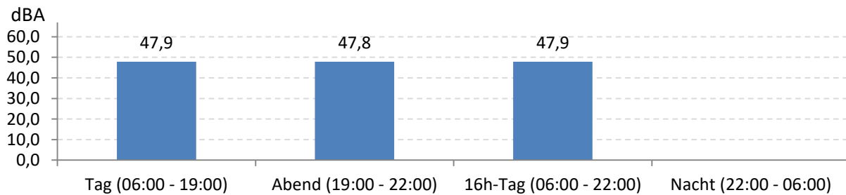
Abb. 7: LEQ bei Pistenbetriebsrichtung "westliche Winde" 552 Stunden im Messzeitraum
