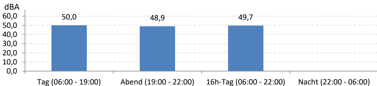
Abb. 8: LEQ bei Pistenbetriebsrichtung "Windstille" 144 Stunden im Messzeitraum
