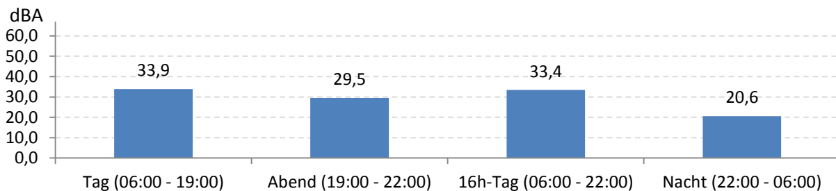
Abb. 8: LEQ bei Pistenbetriebsrichtung "Windstille" 226 Stunden im Messzeitraum
