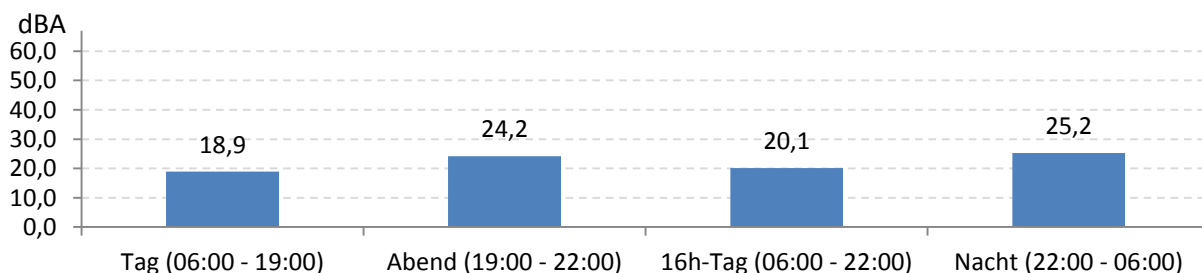
Abb. 9: LEQ bei Pistenbetriebsrichtung "östliche Winde" 259 Stunden im Messzeitraum
