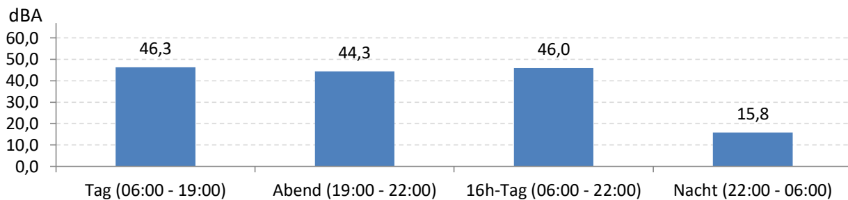
Abb. 6: LEQ für den gesamten Messzeitraum während der Messdauer (Gesamt: 864 Stunden)
