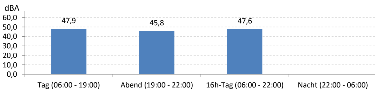
Abb. 8: LEQ bei Pistenbetriebsrichtung "Windstille" 241 Stunden im Messzeitraum
