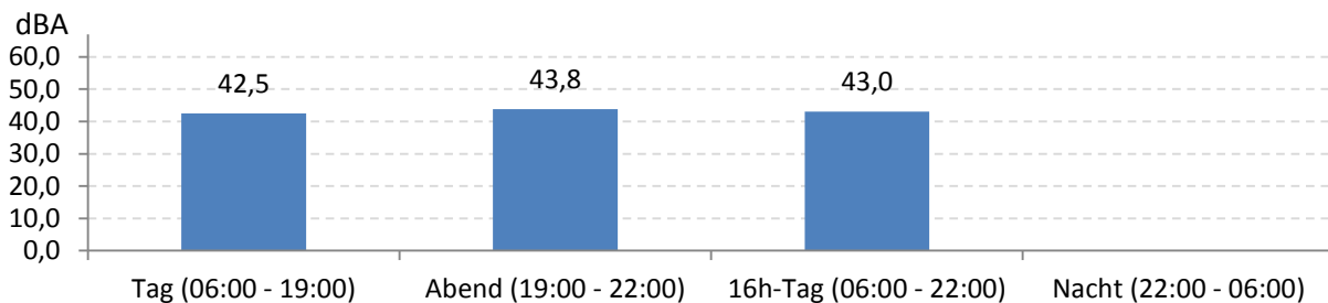
Abb. 8: LEQ bei Pistenbetriebsrichtung "Windstille" 100 Stunden im Messzeitraum
