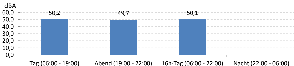
Abb. 9: LEQ bei Pistenbetriebsrichtung "östliche Winde" 260 Stunden im Messzeitraum
