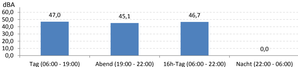
Abb. 6: LEQ für den gesamten Messzeitraum während der Messdauer (Gesamt: 625 Stunden)
