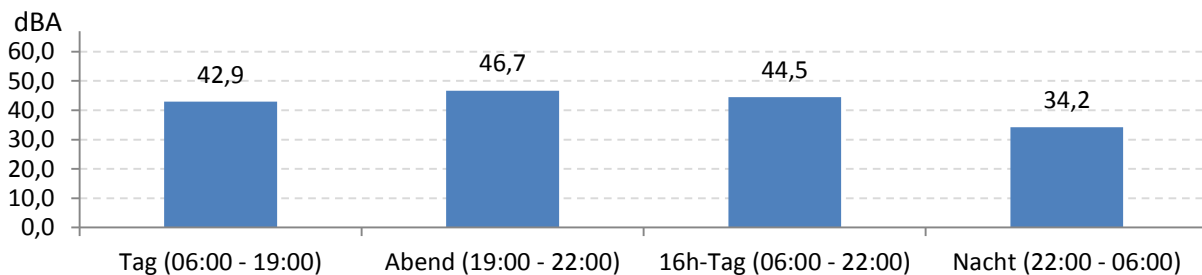
Abb. 8: LEQ bei Pistenbetriebsrichtung "Windstille" 112 Stunden im Messzeitraum
