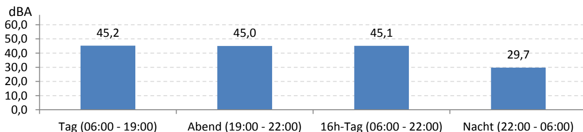
Abb. 9: LEQ bei Pistenbetriebsrichtung "östliche Winde" 284 Stunden im Messzeitraum
