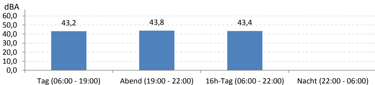
Abb. 8: LEQ bei Pistenbetriebsrichtung "Windstille" 150 Stunden im Messzeitraum
