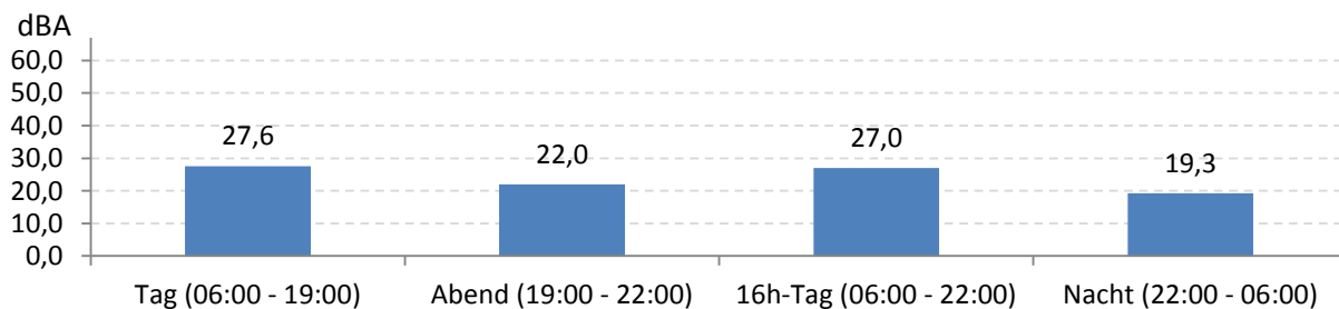
Abb. 7: LEQ bei Pistenbetriebsrichtung "westliche Winde" 471 Stunden im Messzeitraum
