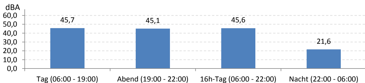
Abb. 9: LEQ bei Pistenbetriebsrichtung "östliche Winde" 99 Stunden im Messzeitraum
