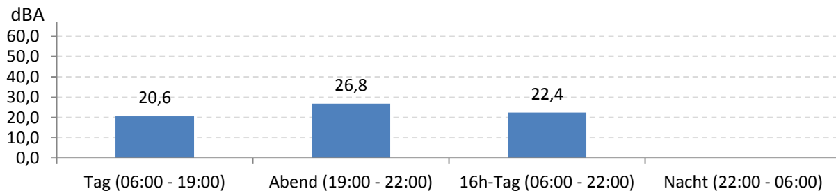
Abb. 7: LEQ bei Pistenbetriebsrichtung "westliche Winde" 414 Stunden im Messzeitraum
