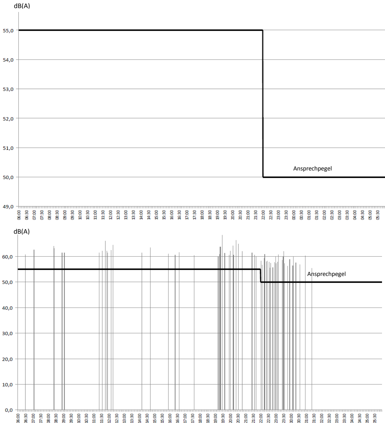
Abb. 12: Verteilung des Maximalpegels bei westlichen Winden
