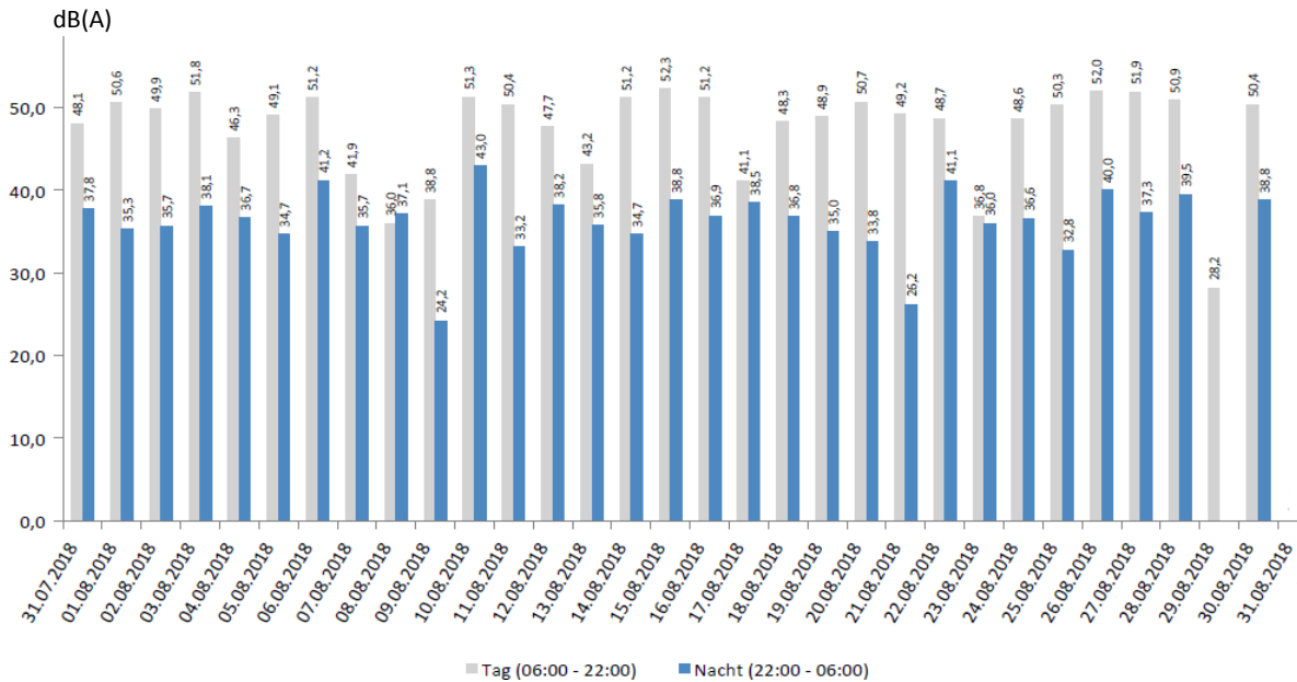
Abb.10: LEQ für Flugverkehr über den Messzeitraum
