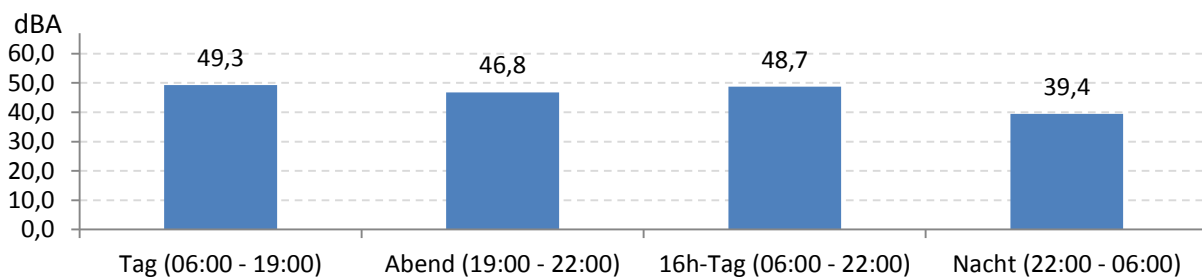
Abb. 8: LEQ bei Pistenbetriebsrichtung "Windstille" 169 Stunden im Messzeitraum
