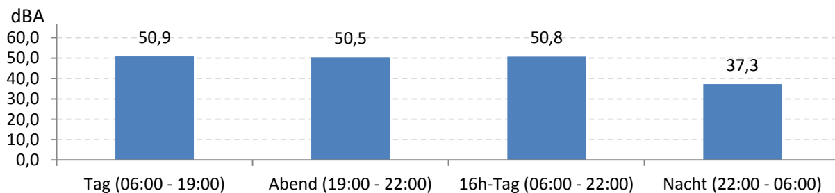
Abb. 7: LEQ bei Pistenbetriebsrichtung "westliche Winde" 501 Stunden im Messzeitraum
