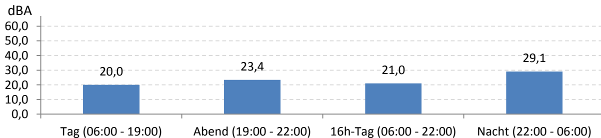
Abb. 7: LEQ bei Pistenbetriebsrichtung "westliche Winde" 595 Stunden im Messzeitraum
