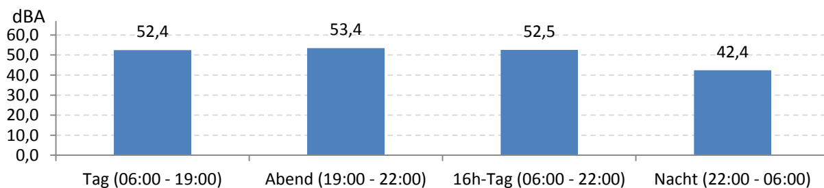
Abb. 9: LEQ bei Pistenbetriebsrichtung "östliche Winde" 71 Stunden im Messzeitraum
