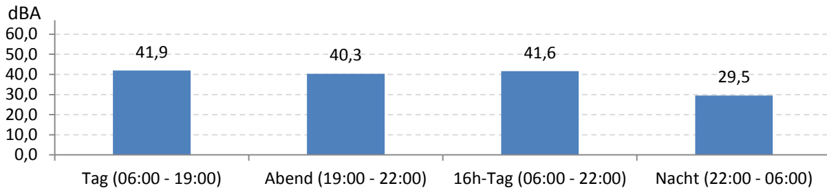
Abb. 6: LEQ für den gesamten Messzeitraum während der Messdauer (Gesamt: 1464 Stunden)
