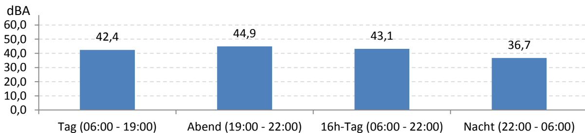
Abb. 8: LEQ bei Pistenbetriebsrichtung "Windstille" 218 Stunden im Messzeitraum
