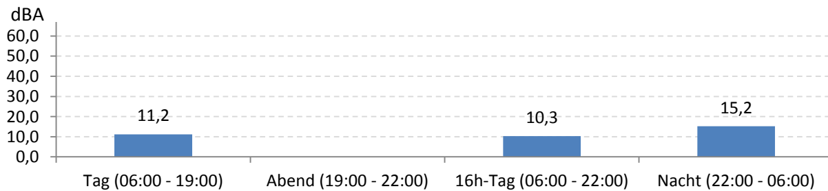
Abb. 7: LEQ bei Pistenbetriebsrichtung "westliche Winde" 1175 Stunden im Messzeitraum
