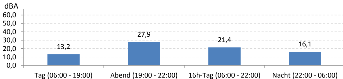
Abb. 7: LEQ bei Pistenbetriebsrichtung "westliche Winde" 375 Stunden im Messzeitraum
