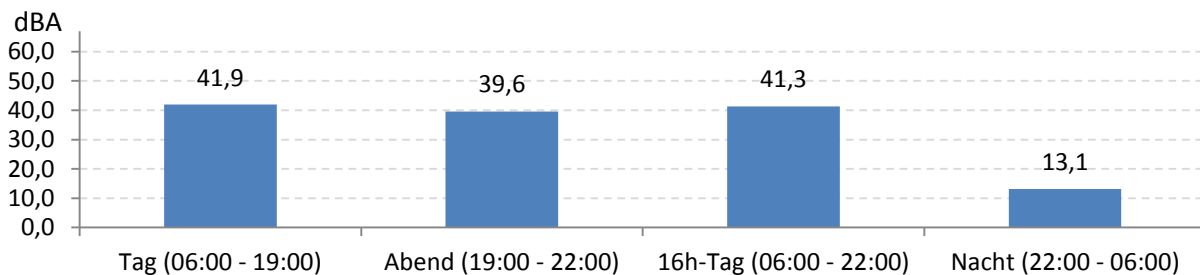
Abb. 8: LEQ bei Pistenbetriebsrichtung "Windstille" 164 Stunden im Messzeitraum
