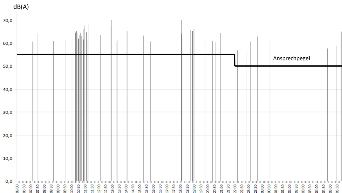
Abb. 13: Verteilung des Maximalpegels bei östlichen Winden
