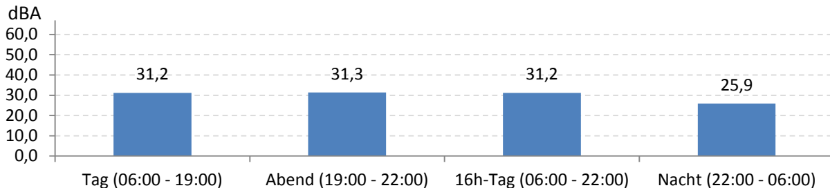
Abb. 6: LEQ für den gesamten Messzeitraum während der Messdauer (Gesamt: 672 Stunden)
