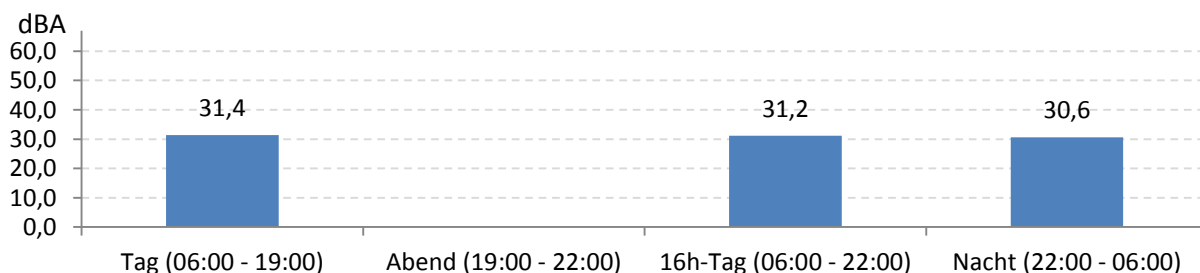
Abb. 9: LEQ bei Pistenbetriebsrichtung "östliche Winde" 156 Stunden im Messzeitraum
