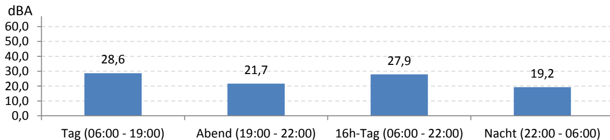
Abb. 7: LEQ bei Pistenbetriebsrichtung "westliche Winde" 354 Stunden im Messzeitraum
