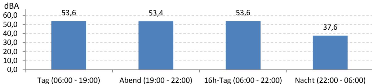
Abb. 6: LEQ für den gesamten Messzeitraum während der Messdauer (Gesamt: 815 Stunden)
