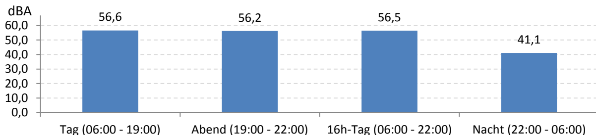
Abb. 8: LEQ bei Pistenbetriebsrichtung "Windstille" 148 Stunden im Messzeitraum
