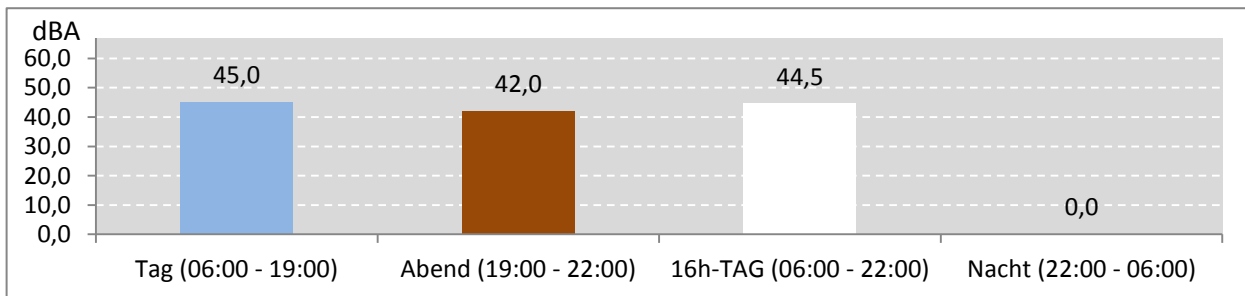
Abb. 9: LEQ bei Pistenbetriebsrichtung "östliche Winde" 77 Stunden im Messzeitraum
