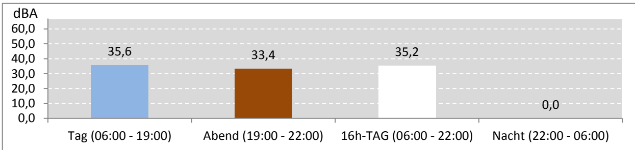
Abb. 6: LEQ für den gesamten Messzeitraum während der Messdauer (Gesamt: 708 Stunden)
