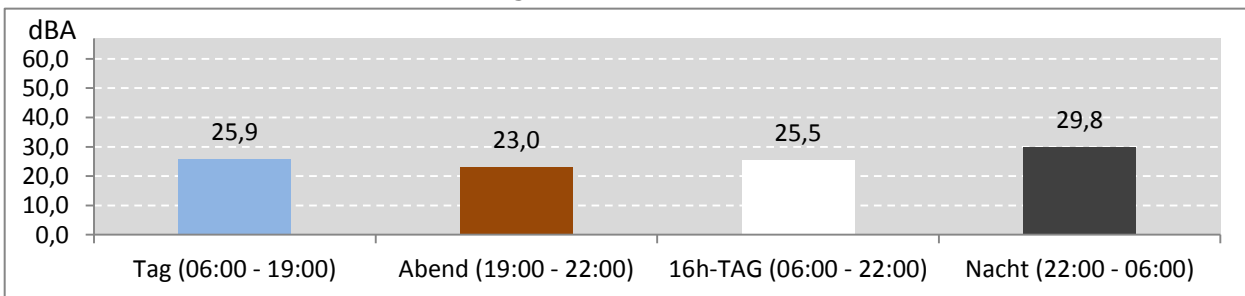
Abb. 8: LEQ bei Pistenbetriebsrichtung "Windstille" 118 Stunden im Messzeitraum
