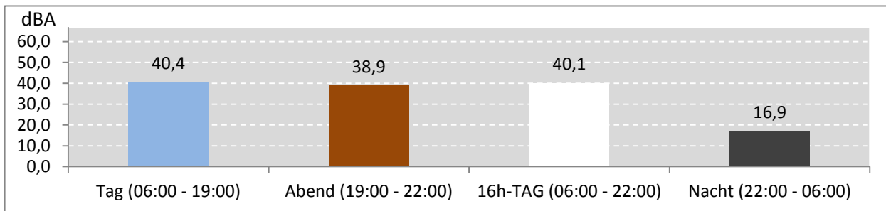
Abb. 7: LEQ bei Pistenbetriebsrichtung "westliche Winde" 322 Stunden im Messzeitraum
