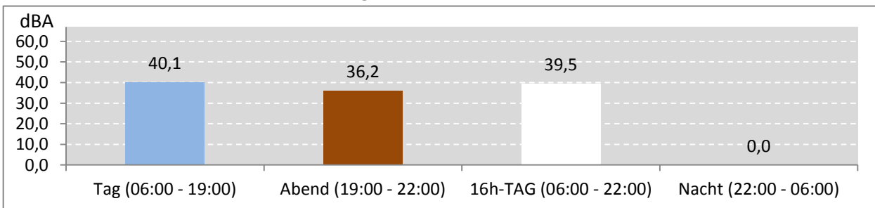
Abb. 8: LEQ bei Pistenbetriebsrichtung "Windstille" 143 Stunden im Messzeitraum
