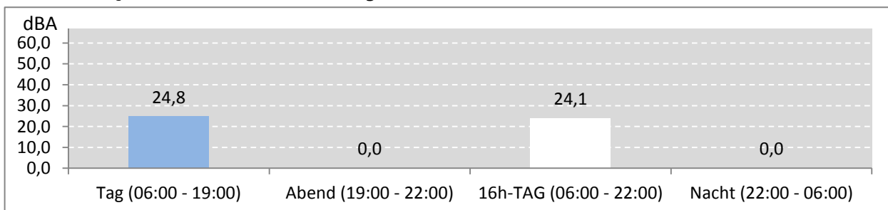
Abb. 9: LEQ bei Pistenbetriebsrichtung "östliche Winde" 64 Stunden im Messzeitraum
