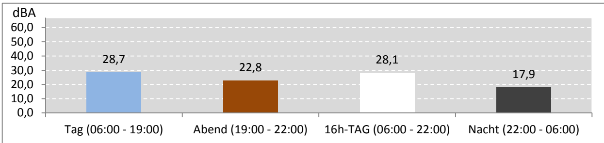
Abb. 6: LEQ für den gesamten Messzeitraum während der Messdauer (Gesamt: 388 Stunden)
