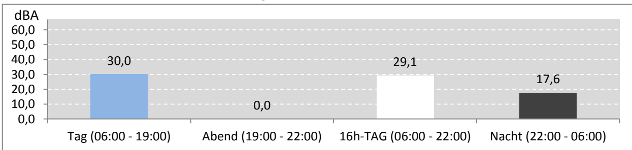
Abb. 8: LEQ bei Pistenbetriebsrichtung "Windstille" 113 Stunden im Messzeitraum
