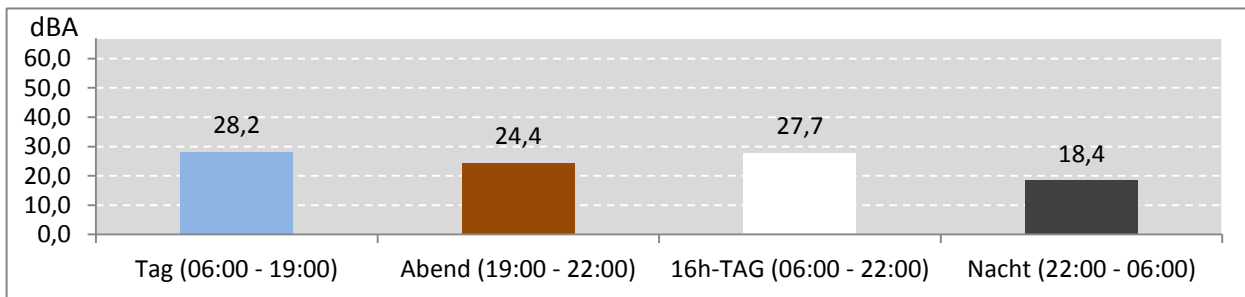
Abb. 7: LEQ bei Pistenbetriebsrichtung "westliche Winde" 260 Stunden im Messzeitraum
