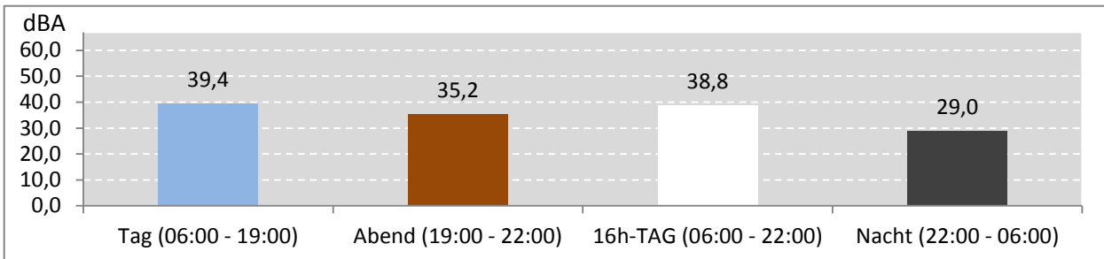
Abb. 6: LEQ für den gesamten Messzeitraum während der Messdauer (Gesamt: 286 Stunden)
