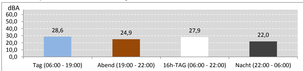
Abb. 9: LEQ bei Pistenbetriebsrichtung "östliche Winde" 51 Stunden im Messzeitraum
