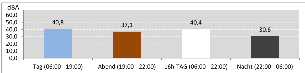
Abb. 7: LEQ bei Pistenbetriebsrichtung "westliche Winde" 195 Stunden im Messzeitraum
