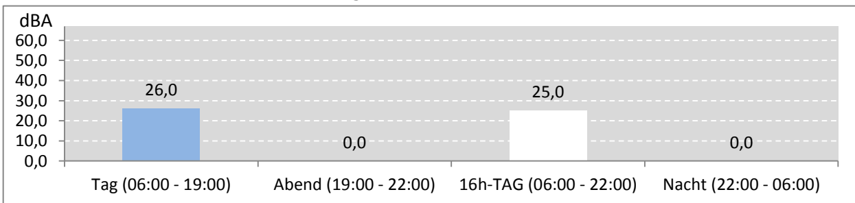
Abb. 8: LEQ bei Pistenbetriebsrichtung "Windstille" 40 Stunden im Messzeitraum
