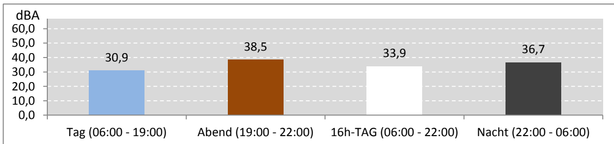
Abb. 9: LEQ bei Pistenbetriebsrichtung "östliche Winde" 119 Stunden im Messzeitraum
