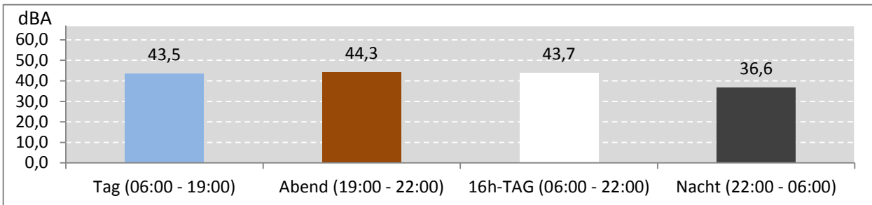
Abb. 6: LEQ für den gesamten Messzeitraum während der Messdauer (Gesamt: 306 Stunden)
