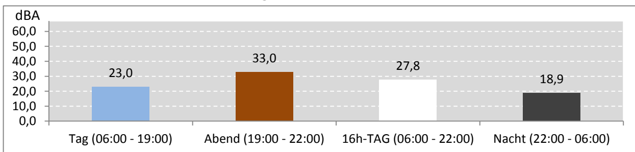
Abb. 7: LEQ bei Pistenbetriebsrichtung "westliche Winde" 168 Stunden im Messzeitraum
