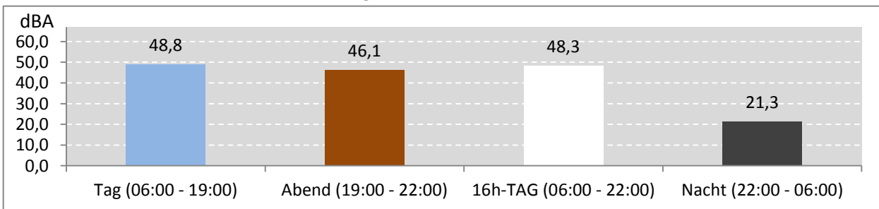
Abb. 8: LEQ bei Pistenbetriebsrichtung "Windstille" 56 Stunden im Messzeitraum
