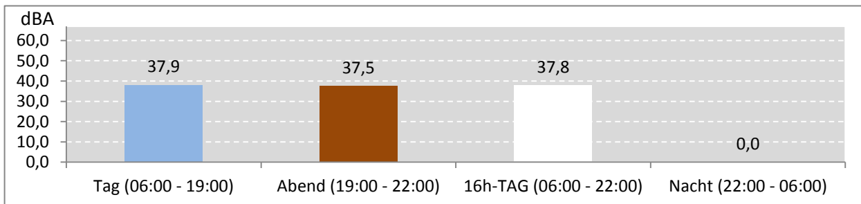
Abb. 7: LEQ bei Pistenbetriebsrichtung "westliche Winde" 177 Stunden im Messzeitraum
