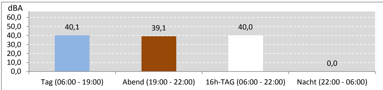
Abb. 6: LEQ für den gesamten Messzeitraum während der Messdauer (Gesamt: 313 Stunden)
