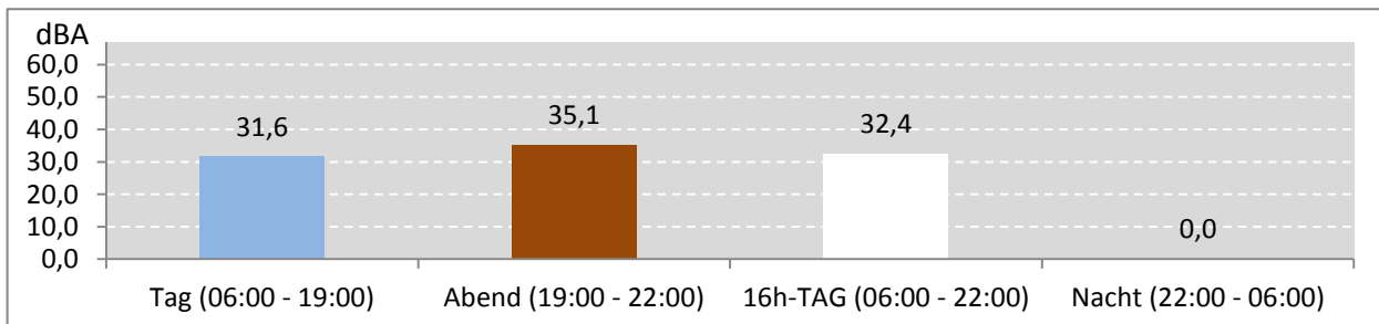
Abb. 9: LEQ bei Pistenbetriebsrichtung "östliche Winde" 50 Stunden im Messzeitraum
