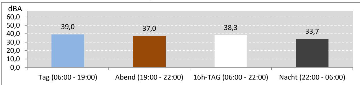
Abb. 8: LEQ bei Pistenbetriebsrichtung "Windstille" 76 Stunden im Messzeitraum
