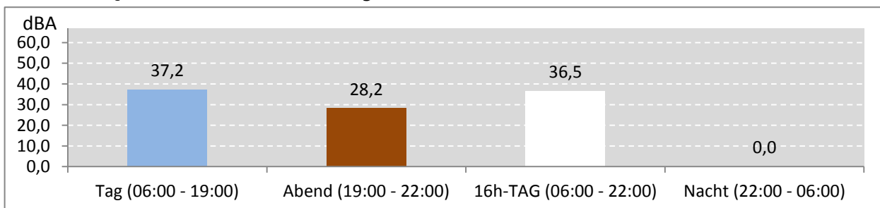
Abb. 9: LEQ bei Pistenbetriebsrichtung "östliche Winde" 54 Stunden im Messzeitraum
