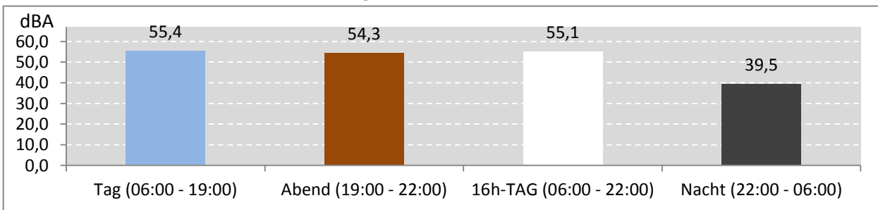
Abb. 8: LEQ bei Pistenbetriebsrichtung "Windstille" 53 Stunden im Messzeitraum
