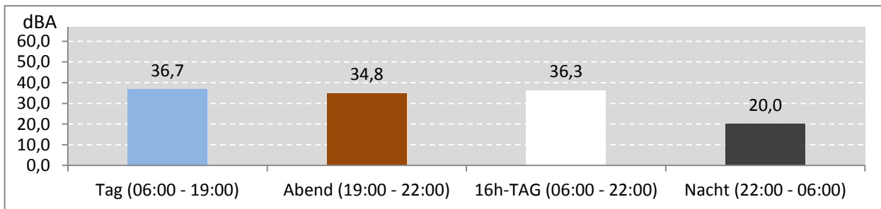
Abb. 9: LEQ bei Pistenbetriebsrichtung "östliche Winde" 94 Stunden im Messzeitraum
