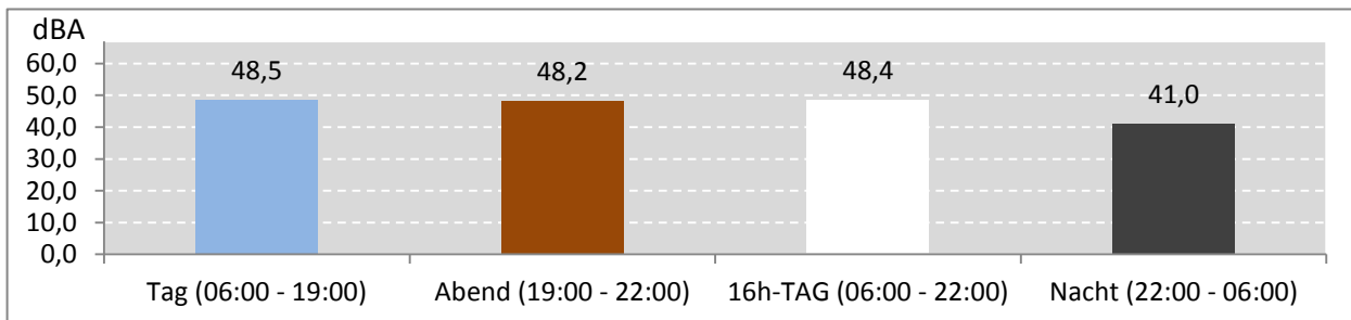
Abb. 7: LEQ bei Pistenbetriebsrichtung "westliche Winde" 271 Stunden im Messzeitraum
