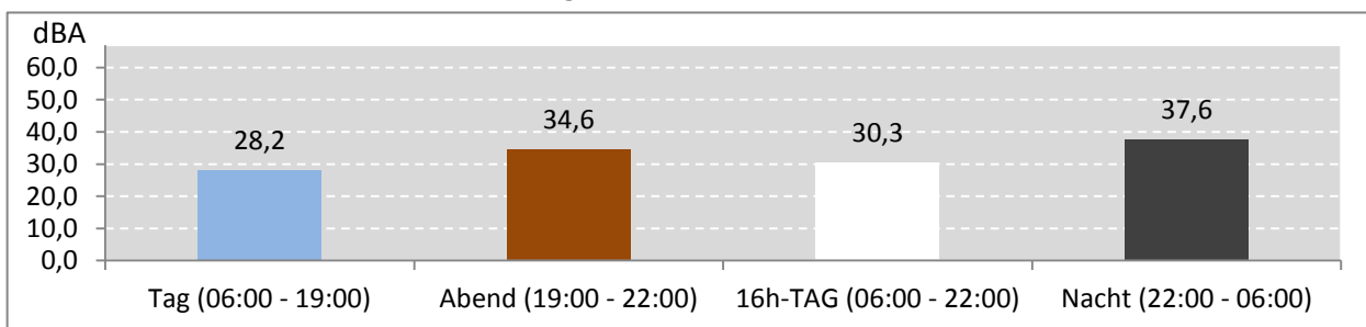
Abb. 7: LEQ bei Pistenbetriebsrichtung "westliche Winde" 333 Stunden im Messzeitraum
