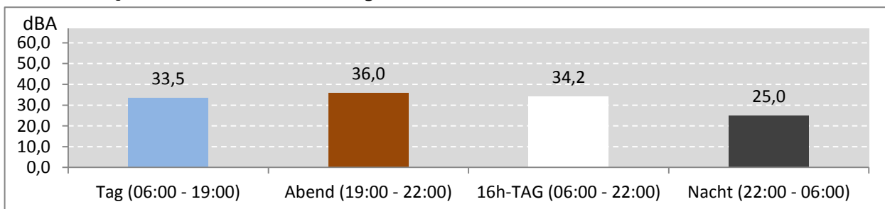
Abb. 9: LEQ bei Pistenbetriebsrichtung "östliche Winde" 58 Stunden im Messzeitraum
