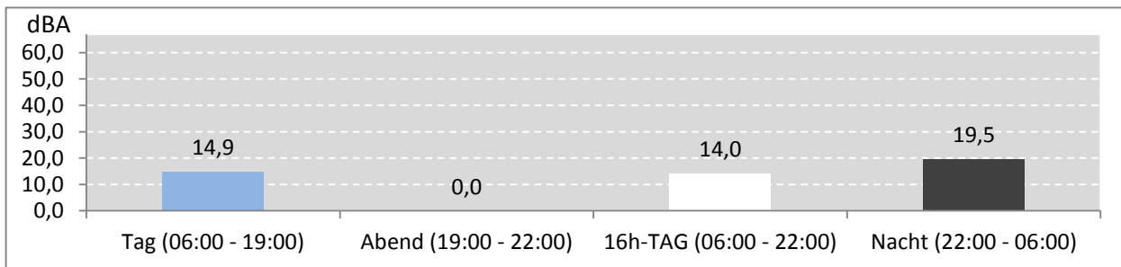
Abb. 7: LEQ bei Pistenbetriebsrichtung "westliche Winde" 297 Stunden im Messzeitraum
