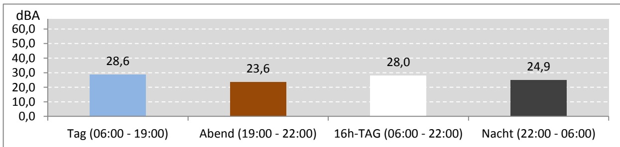
Abb. 9: LEQ bei Pistenbetriebsrichtung "östliche Winde" 79 Stunden im Messzeitraum
