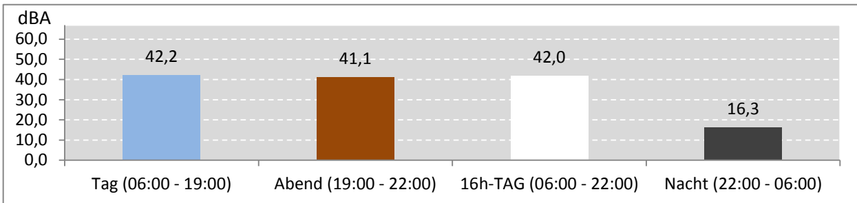
Abb. 6: LEQ für den gesamten Messzeitraum während der Messdauer (Gesamt: 507 Stunden)
