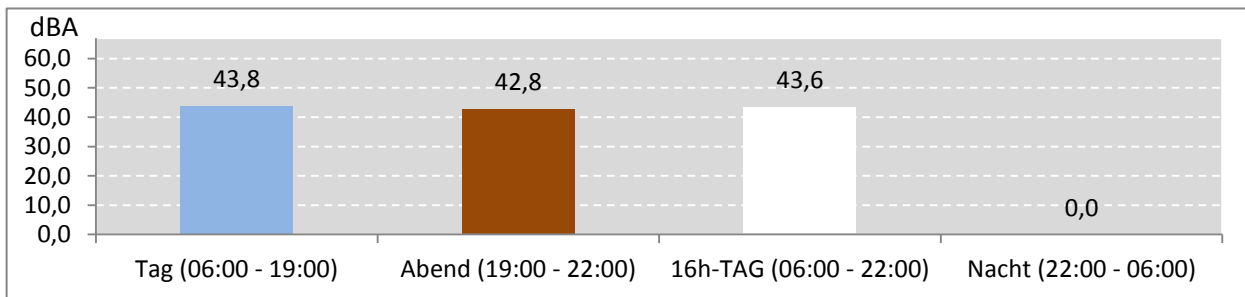
Abb. 7: LEQ bei Pistenbetriebsrichtung "westliche Winde" 326 Stunden im Messzeitraum
