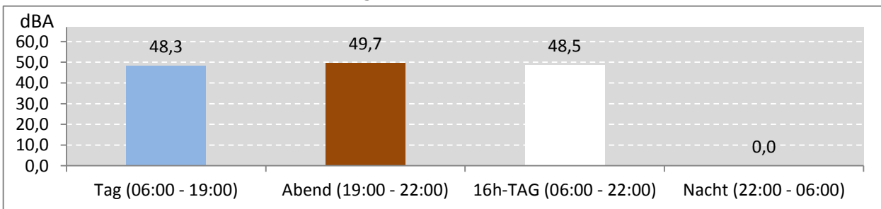
Abb. 8: LEQ bei Pistenbetriebsrichtung "Windstille" 46 Stunden im Messzeitraum
