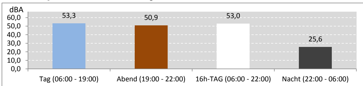
Abb. 9: LEQ bei Pistenbetriebsrichtung "östliche Winde" 200 Stunden im Messzeitraum
