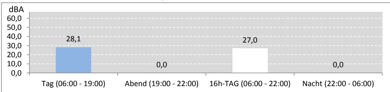
Abb. 8: LEQ bei Pistenbetriebsrichtung "Windstille" 155 Stunden im Messzeitraum
