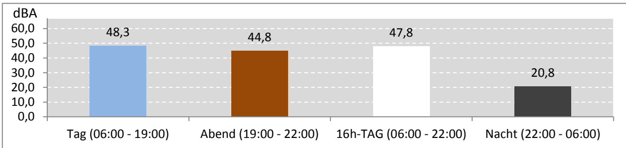
Abb. 6: LEQ für den gesamten Messzeitraum während der Messdauer (Gesamt: 638 Stunden)
