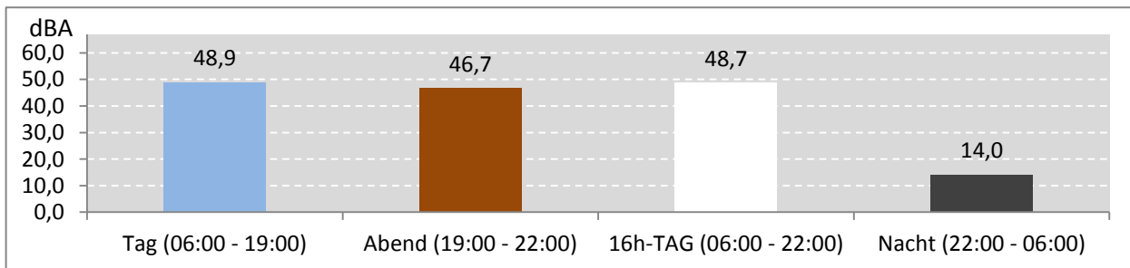
Abb. 9: LEQ bei Pistenbetriebsrichtung "östliche Winde" 179 Stunden im Messzeitraum
