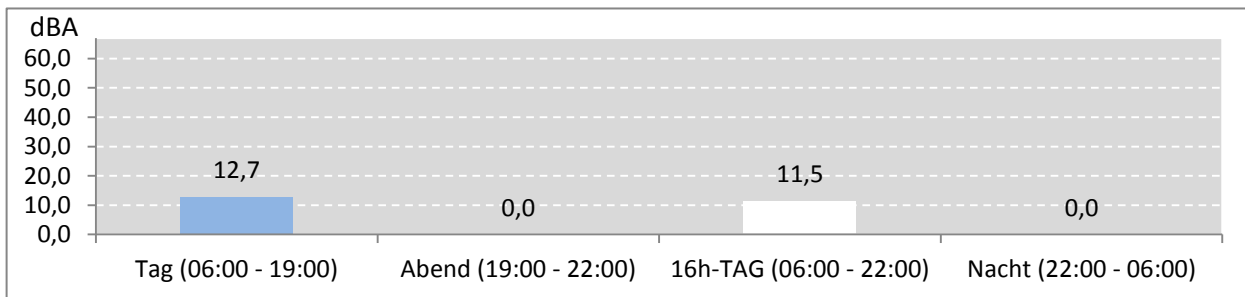
Abb. 7: LEQ bei Pistenbetriebsrichtung "westliche Winde" 263 Stunden im Messzeitraum
