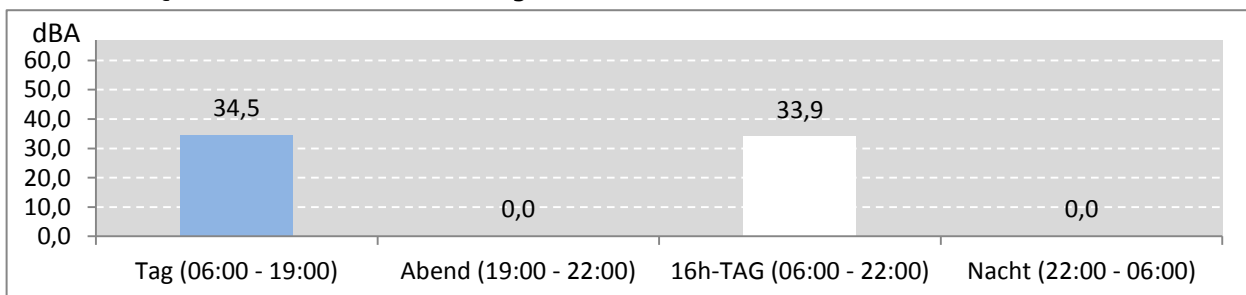
Abb. 9: LEQ bei Pistenbetriebsrichtung "östliche Winde" 89 Stunden im Messzeitraum
