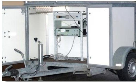
Abb. 4: Messgerät und Modemeinheit:
