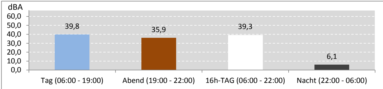
Abb. 6: LEQ für den gesamten Messzeitraum während der Messdauer (Gesamt: 420 Stunden)
