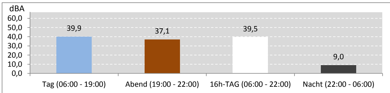
Abb. 7: LEQ bei Pistenbetriebsrichtung "westliche Winde" 223 Stunden im Messzeitraum
