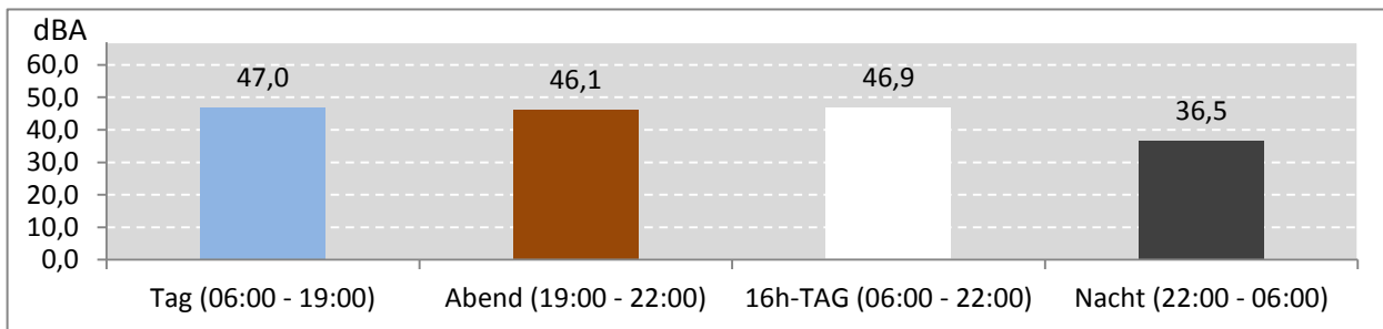
Abb. 7: LEQ bei Pistenbetriebsrichtung "westliche Winde" 314 Stunden im Messzeitraum
