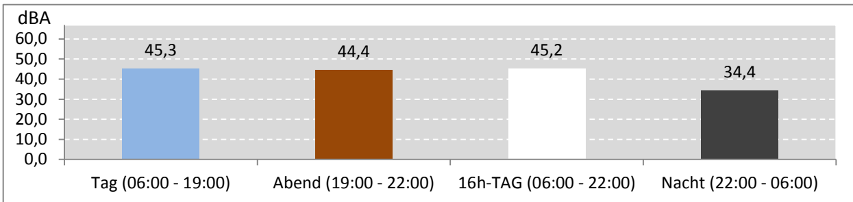
Abb. 6: LEQ für den gesamten Messzeitraum während der Messdauer (Gesamt: 494 Stunden)
