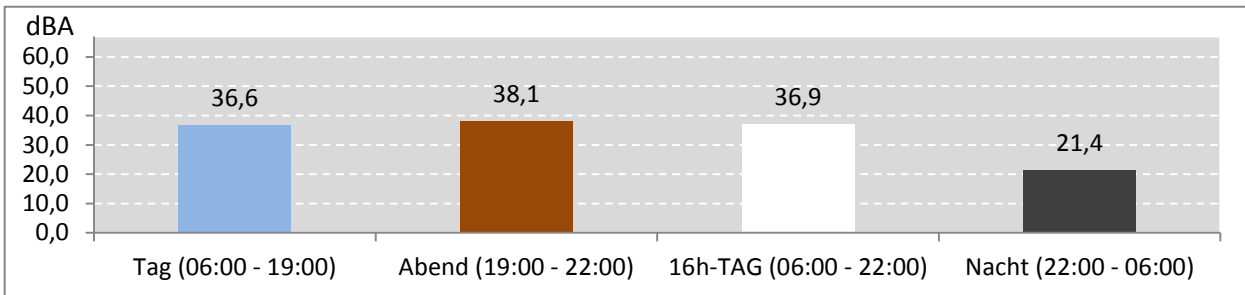
Abb. 6: LEQ für den gesamten Messzeitraum während der Messdauer (Gesamt: 489 Stunden)
