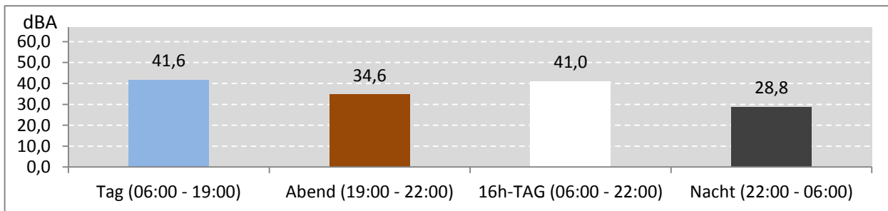
Abb. 9: LEQ bei Pistenbetriebsrichtung "östliche Winde" 61 Stunden im Messzeitraum
