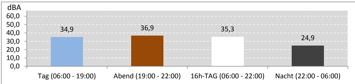
Abb. 6: LEQ für den gesamten Messzeitraum während der Messdauer (Gesamt: 525 Stunden)
