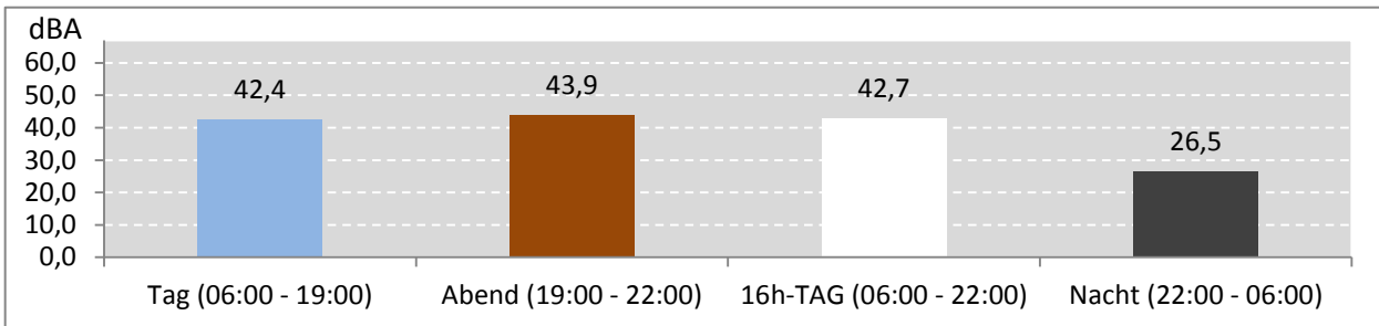
Abb. 6: LEQ für den gesamten Messzeitraum während der Messdauer (Gesamt: 361 Stunden)
