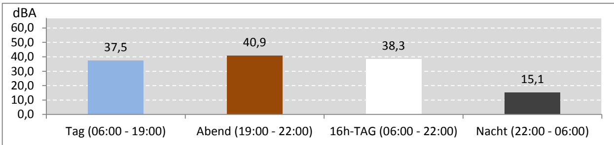
Abb. 6: LEQ für den gesamten Messzeitraum während der Messdauer (Gesamt: 454 Stunden)
