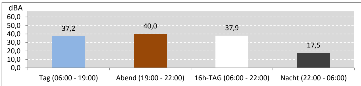
Abb. 7: LEQ bei Pistenbetriebsrichtung "westliche Winde" 290 Stunden im Messzeitraum
