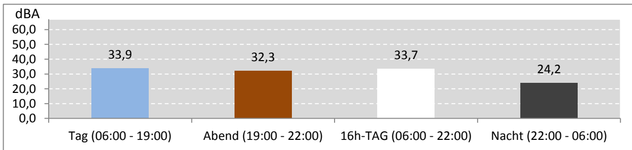
Abb. 7: LEQ bei Pistenbetriebsrichtung "westliche Winde" 308 Stunden im Messzeitraum
