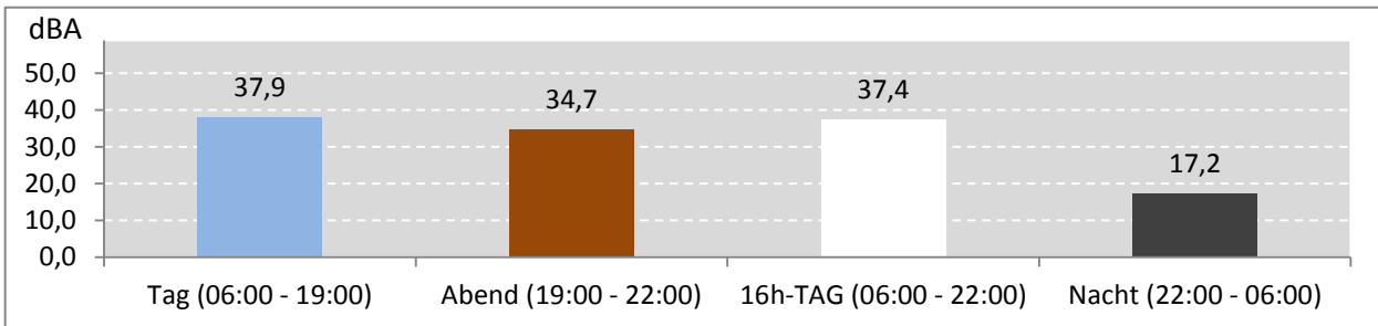
Abb. 6: LEQ für den gesamten Messzeitraum während der Messdauer (Gesamt: 389 Stunden)
