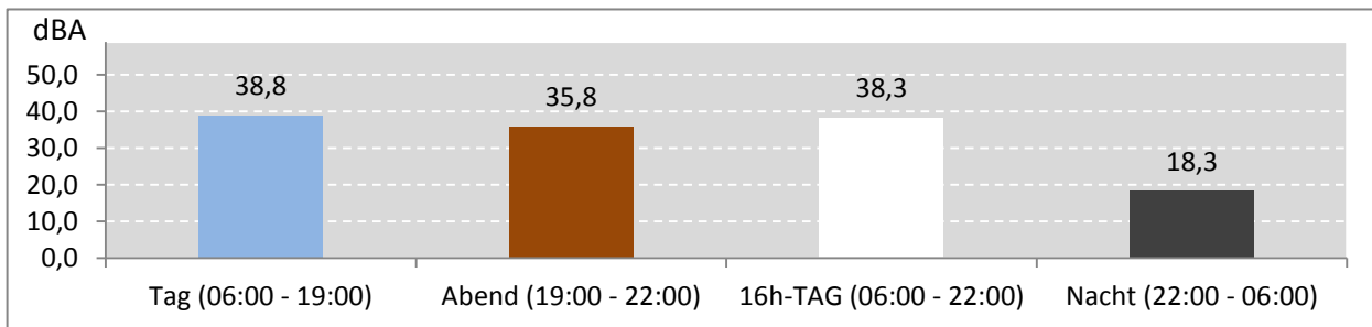
Abb. 7: LEQ bei Pistenbetriebsrichtung "westliche Winde" 232 Stunden im Messzeitraum
