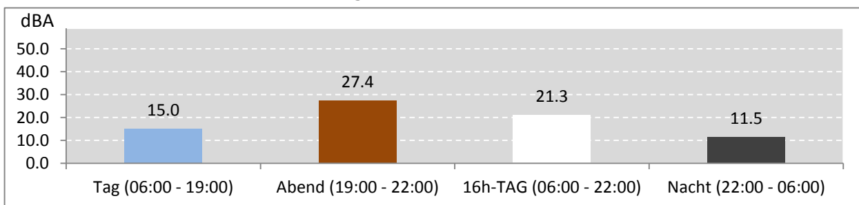
Abb. 7: LEQ bei Pistenbetriebsrichtung "westliche Winde" 240 Stunden im Messzeitraum
