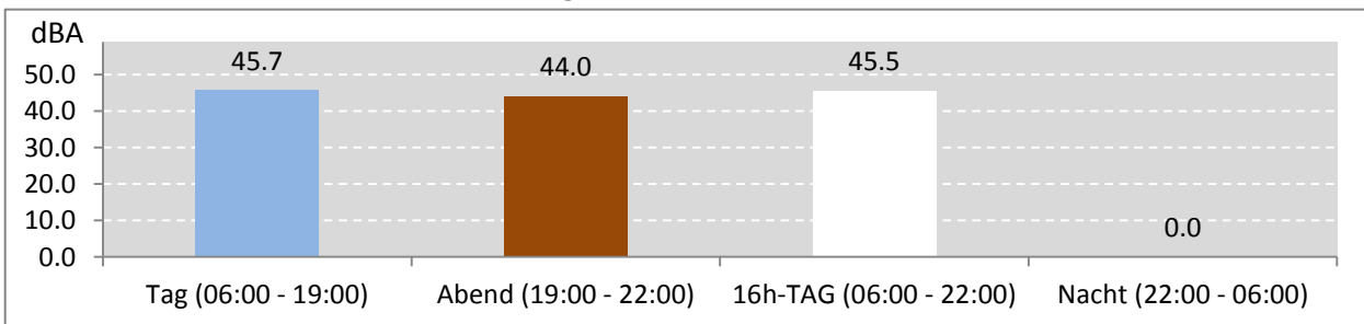
Abb. 8: LEQ bei Pistenbetriebsrichtung "Windstille" 85 Stunden im Messzeitraum
