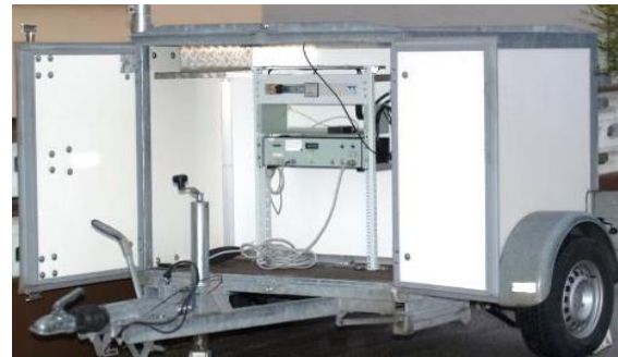
Abb. 4: Messgerät und Modemeinheit:
