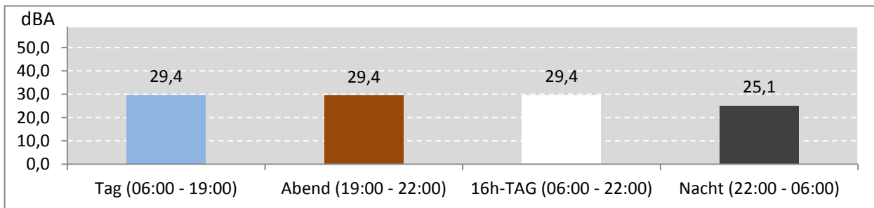
Abb. 7: LEQ bei Pistenbetriebsrichtung "westliche Winde" 312 Stunden im Messzeitraum
