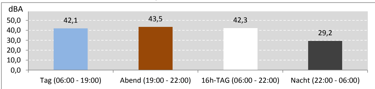
Abb. 8: LEQ bei Pistenbetriebsrichtung "Windstille" 111 Stunden im Messzeitraum
