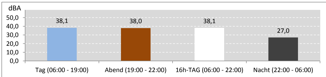
Abb. 9: LEQ bei Pistenbetriebsrichtung "östliche Winde" 133 Stunden im Messzeitraum
