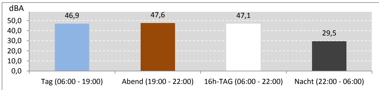
Abb. 7: LEQ bei Pistenbetriebsrichtung "westliche Winde" 244 Stunden im Messzeitraum
